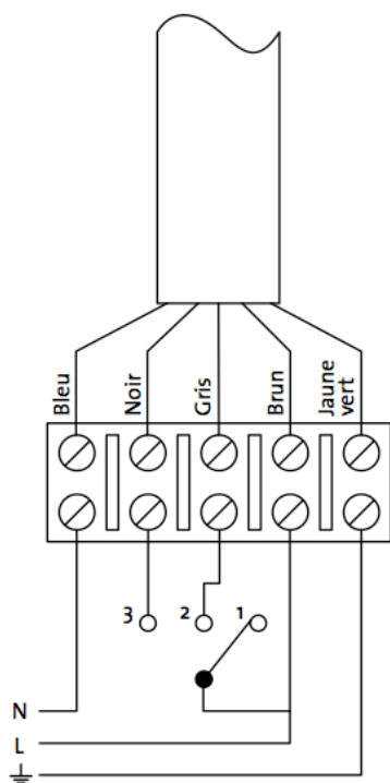
Ventilateur de toiture type CVD
