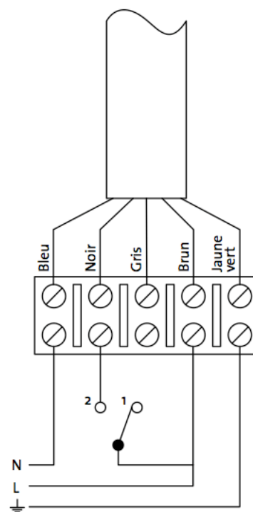
Ventilateur de toiture type CVD
