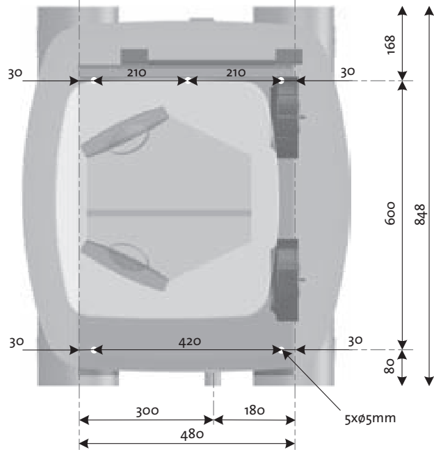
Montage miroité
