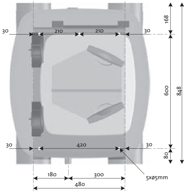
Montage standard
