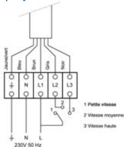
Schéma de principe RS 3
